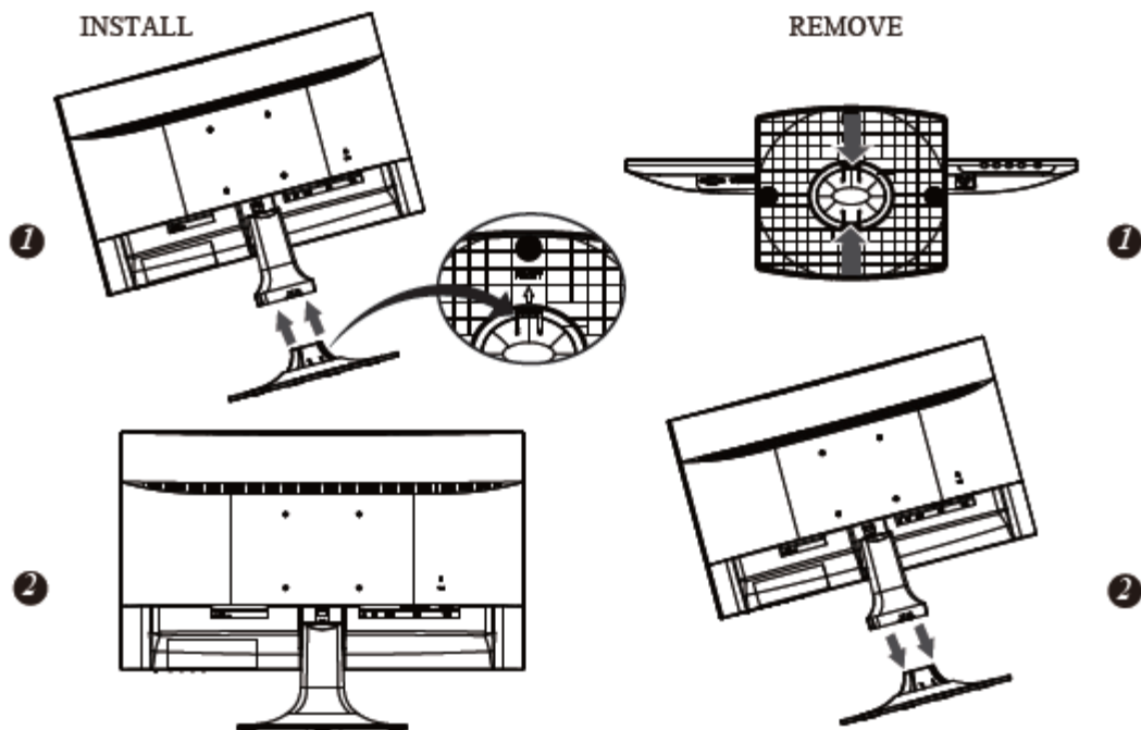
ABBILDUNG 1. INSTALLIEREN UND ENTFERNEN DES STÄNDERS
