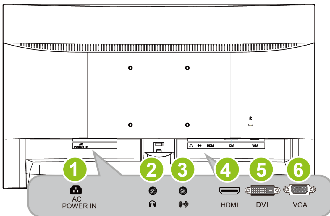
ABBILDUNG 2. ANSCHLISSEN AN EINEN PC
